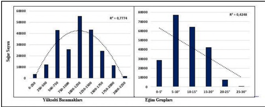
Şekil 5: Kahramanmaraş'ta büyükbaş hayvan sayılarının yükselti ve eğim faktörleri ile ilişkileri
