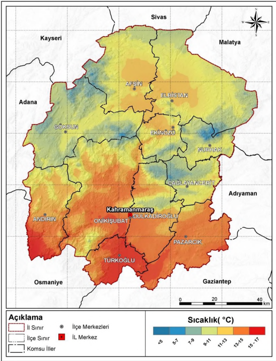
Şekil 2. Kahramanmaraş ili sıcaklık Haritası.
