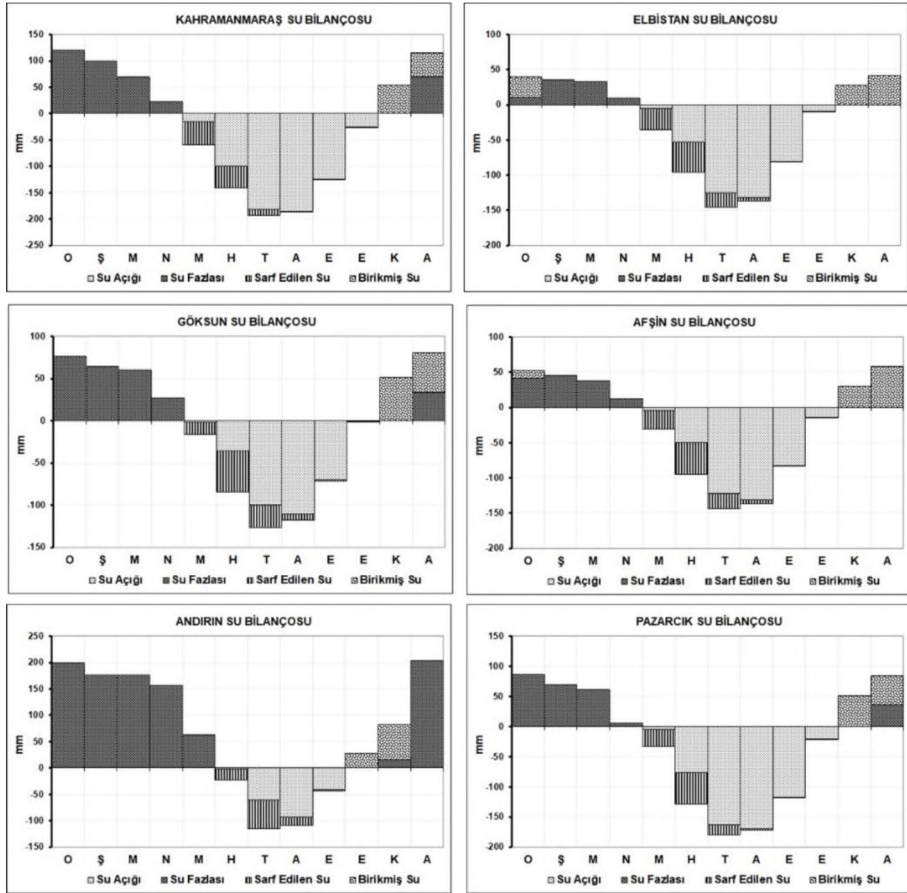
Şekil 4. Thornthwaite metoduna göre çalışma alanındaki istasyonların su bilançoları.
