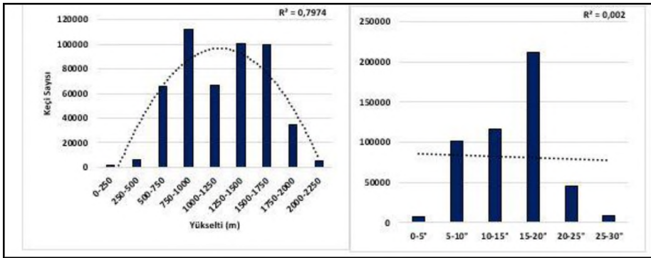
Şekil 7: Kahramanmaraş'ta keçi sayılarının yükselti ve eğim faktörleri ile ilişkileri
