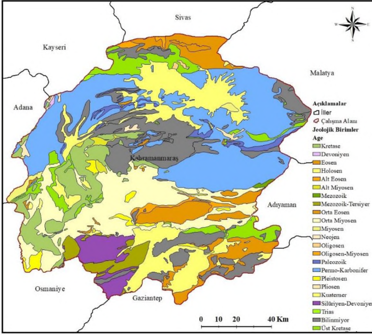
Şekil 3. Çalışma Alanının Jeoloji Haritası.
