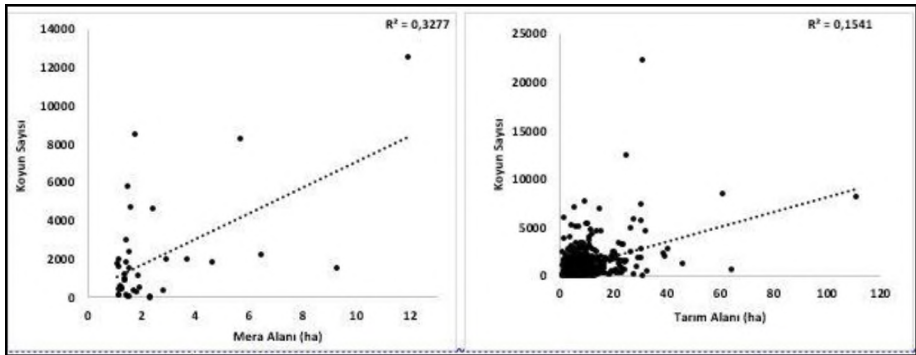
Şekil 10: Kahramanmaraş'ta koyun sayılarının mera ve tarım alanları ile ilişkileri
