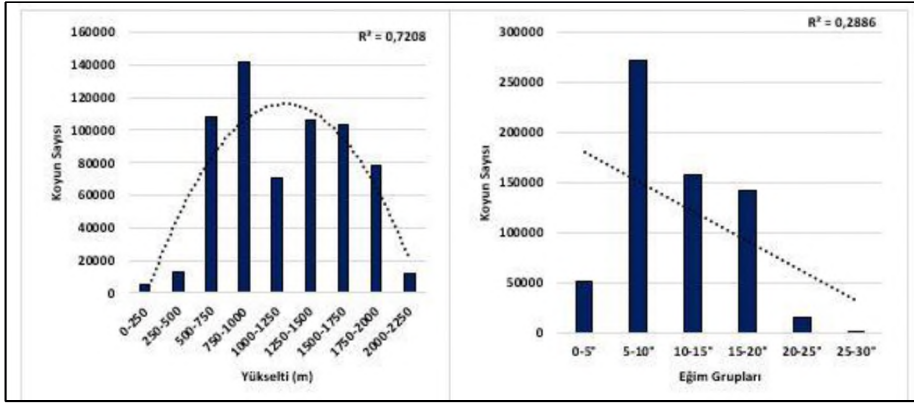
Şekil 6: Kahramanmaraş'ta koyun sayılarının yükselti ve eğim faktörleri ile ilişkileri
