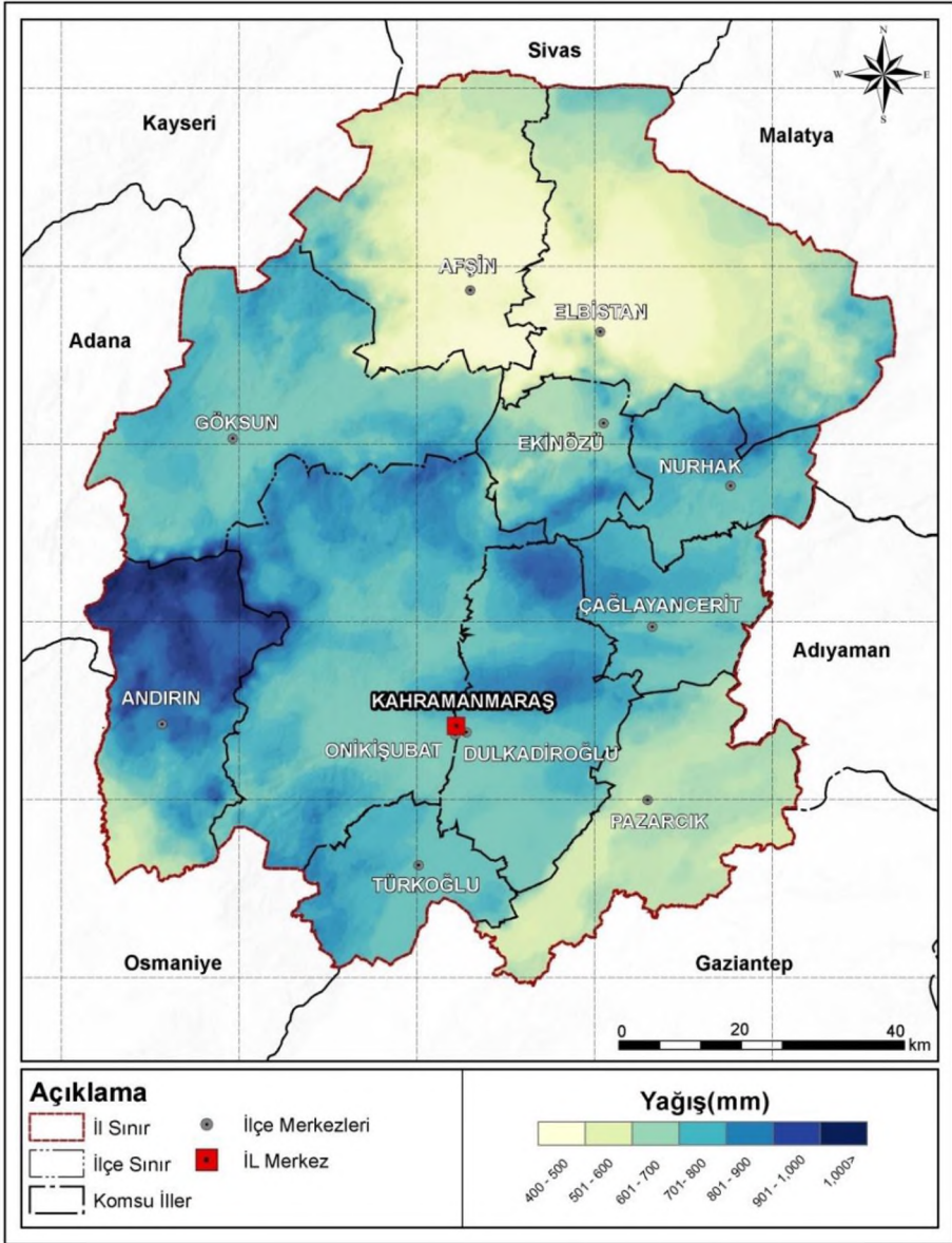
Şekil 3. Kahramanmaraş ili yağış Haritası.
