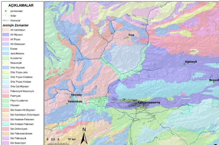
Şekil 3: Kahramanmaraş'ın Jeoloji Haritası
