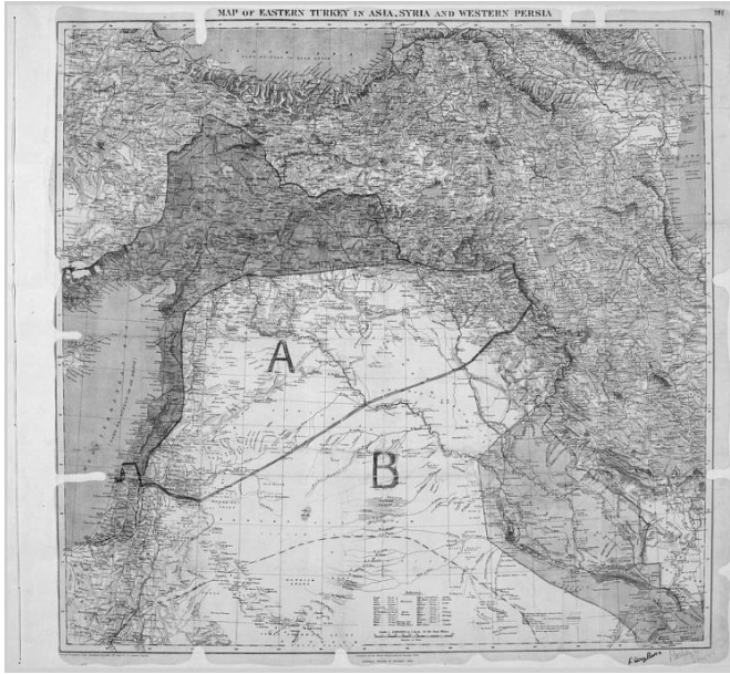
Şekil 1: 1916 yılında imzalanmış Skyes-Picot Anlaşmasına göre Ortadoğu ve Kilikya
