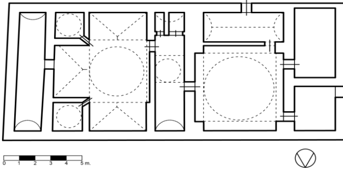
Çizim 1: Uzunluk Hamamı plânı (V. Soğancı'dan işlenerek).
